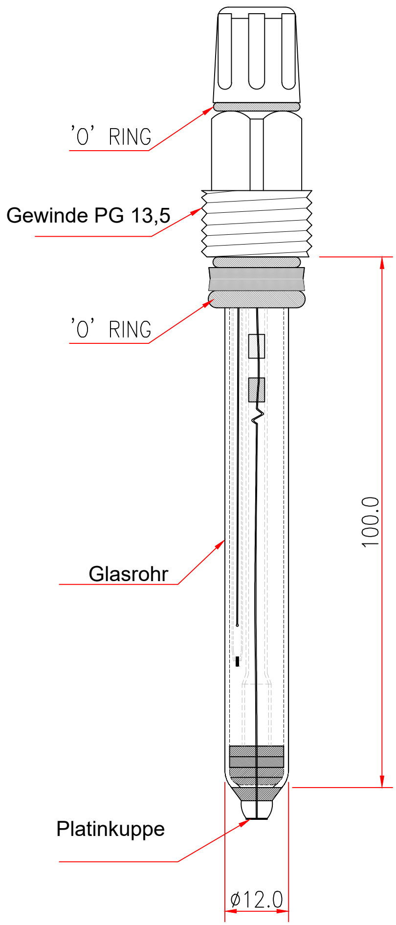
Redoxelektrode PBSIGK2-100
